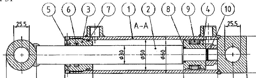
Zylinder 50/30-150
