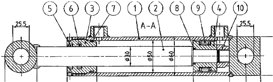
Zylinder 50/30-150
