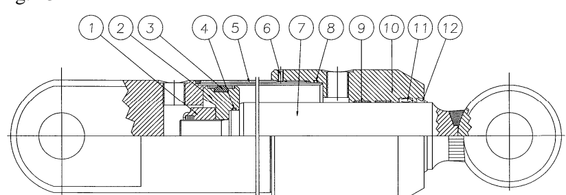
Zylinder 80/50-350
